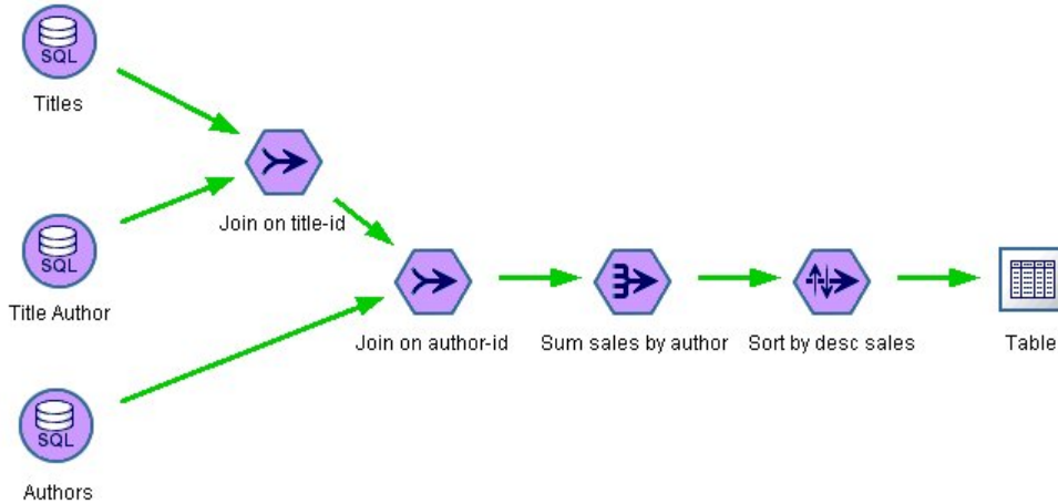
Figura 3. Ruta optimizada con nodos púrpura que indica puntos de retrotracción SQL (operaciones llevadas a cabo en la base de datos)
